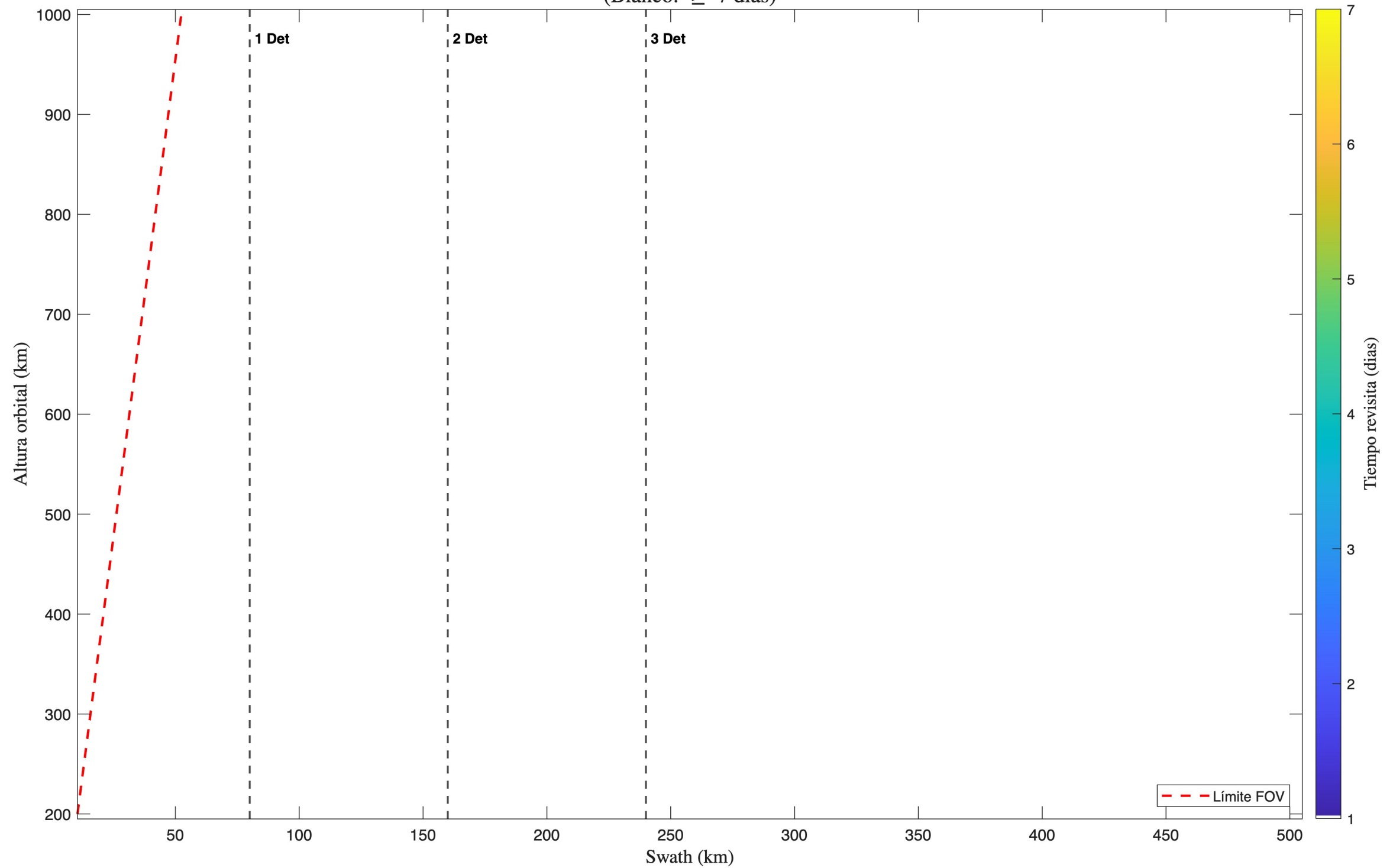
Tiempo Revisita - 2 Satellite(s); 1 Telescopio(s): Cassegrain; Detector 3 (Blanco: \geq 7 días)
